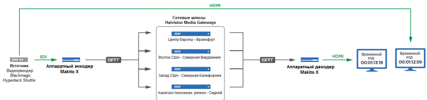
Рисунок 9: Тестовая система с использованием аппаратных энкодеров и декодеров Makito X
